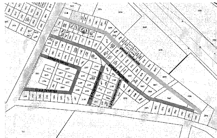
Схема элементов улично-дорожной сети в деревне Ямны муниципального образования город Тула
